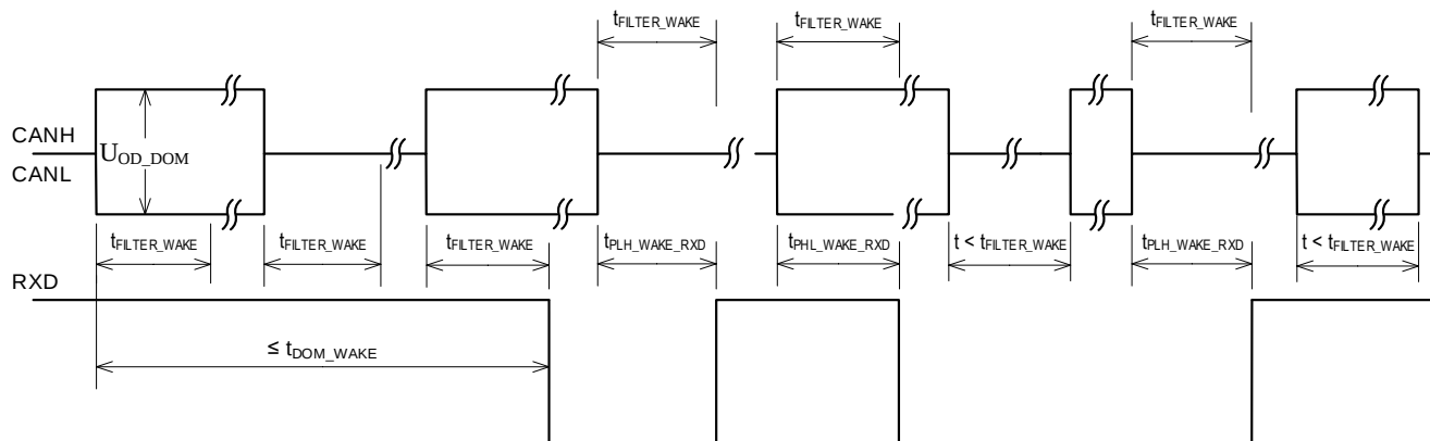
Рисунок 7 – Временная диаграмма приема паттерна wake-up и фильтрации помех на шине после пробуждения
